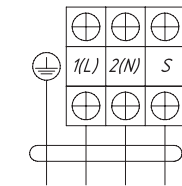
Клеммный терминал внутреннего блока
