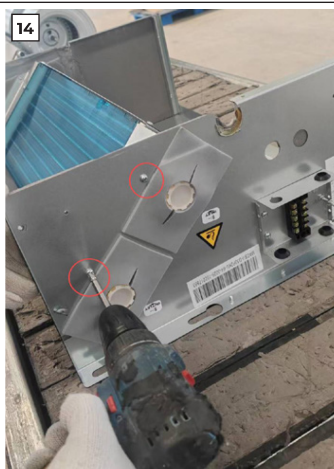
Открутите винты крепления боковых панелей, рис. 14-15
